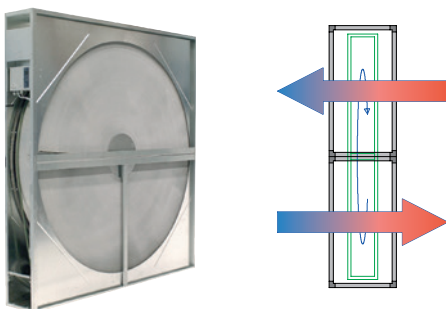
Warmtewiel
