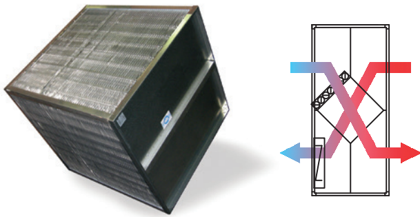
Kruisstroom platenwarmtewisselaar
